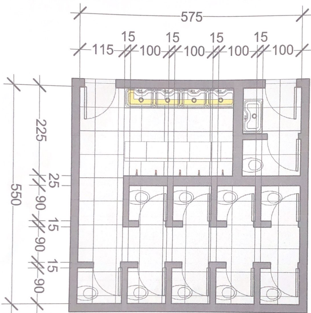
پلان تشنابهای دفتر مرکزی
